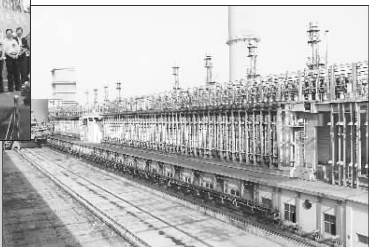
▶佳华公司6.25米捣固焦炉和SCP一体机
